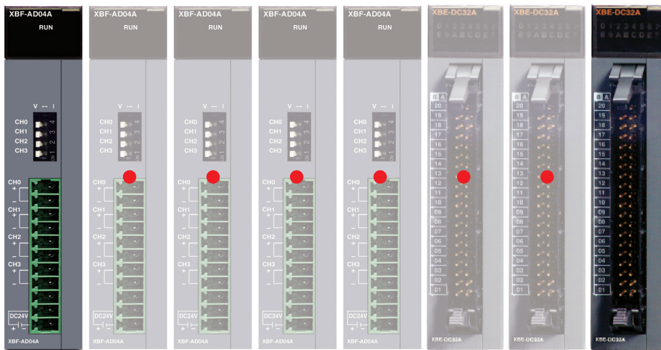
Moduły szybkiej komunikacji + podstawowe moduły rozszerzeń: maks. 10 rozszerzeń
