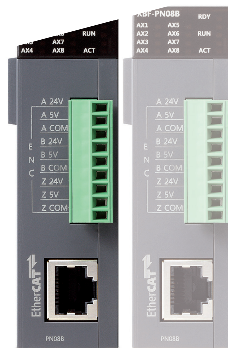
Moduł szybkiej komunikacji: maks. 2 rozszerzenia
